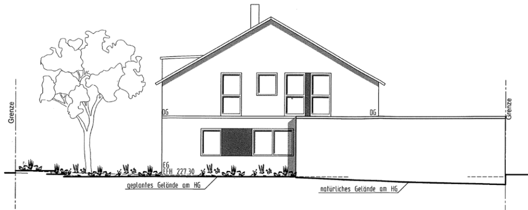
Ostansicht 1:100
