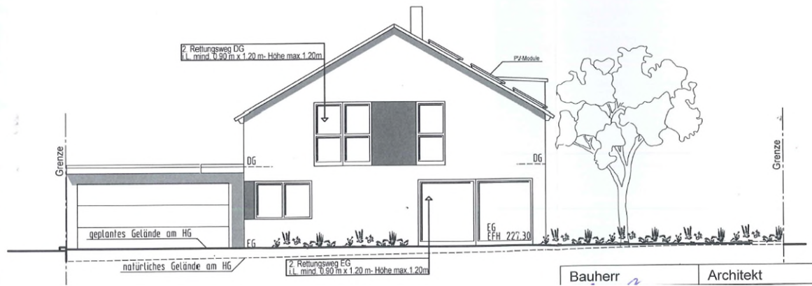
Westansicht 1:100
